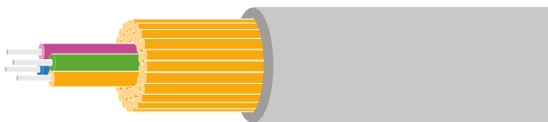
Querschnitt Mehrfasermodell
